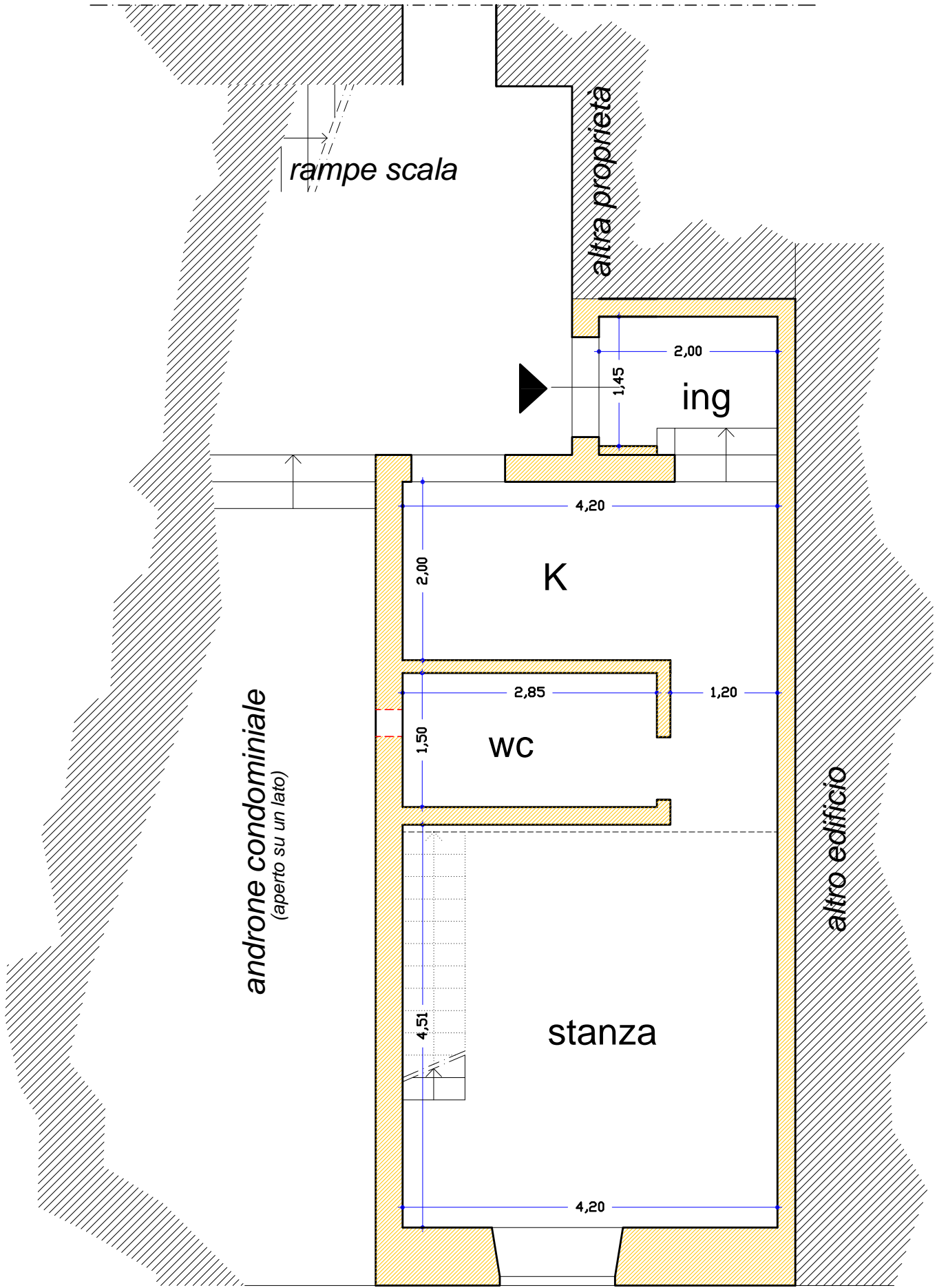
pianta piano rialzato
