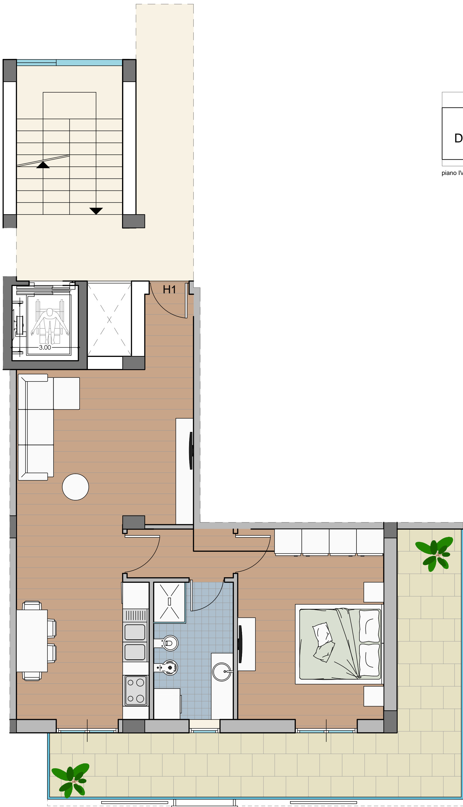
pianta arredata tipologia H1 piano IV scala 1:50
